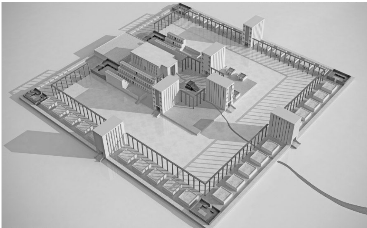
Fig. 6 Model van het heilig Tempelgebied met in het midden daarvan het brandofferaltaar. Let op de hoge poortgebouwen, de enige hoogtemaat die gegeven is, en de treden die de gradatie in heiligheid benadrukken. Door Bibliaprints.
